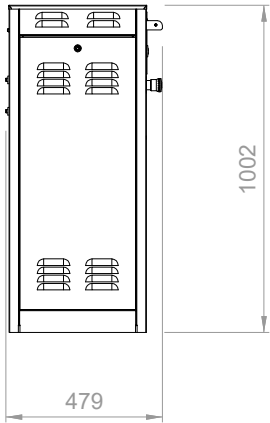
СБОКУ
