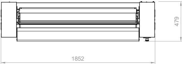
СВЕРХУ
