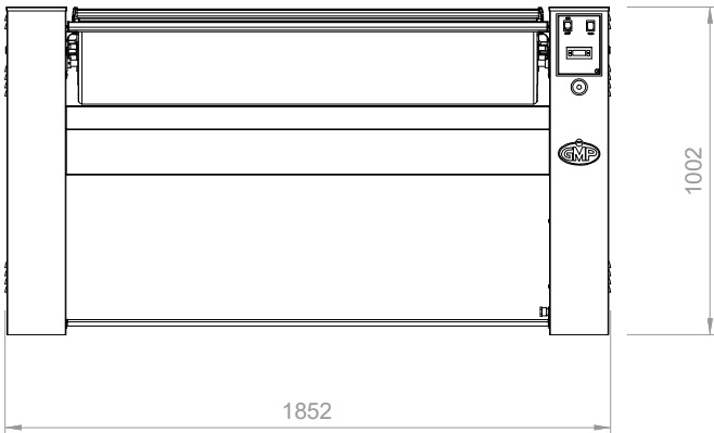
VUE FRONTALE
